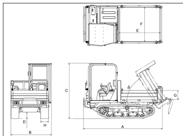
C30R-2B
